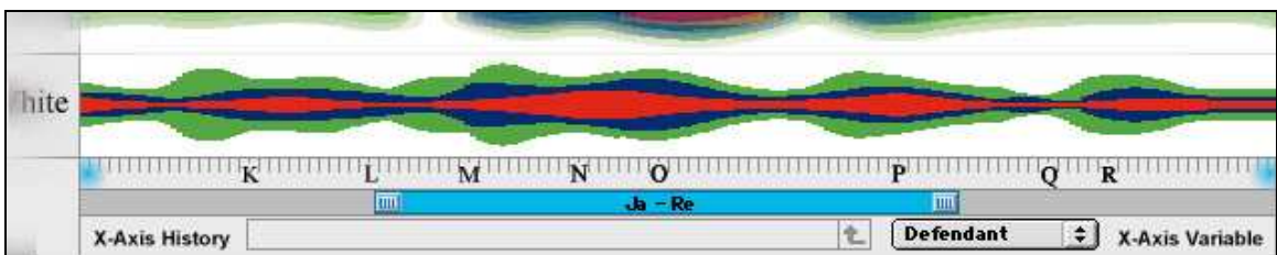
Figure5d:ManagingOvercrowdedAxes:Scroll/Zoom( Sketch)
